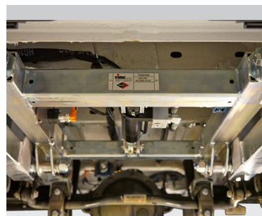
Hydraulische Achsblockierung
